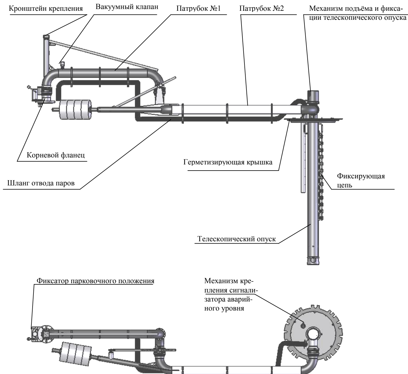
Рис. 1. Конструкция стояка верхнего налива ОСН-СВН-100-У-3-4-НН.
